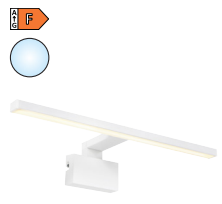
Marlee 50 2310301001 White | Metal LED Module 8,9W | 800lm | 4000K H: 9,6 cm | W: 50 cm | L: 50 cm
