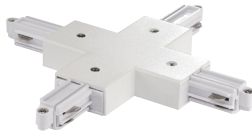
Link X-Connector 86079901 White | Plastic Max. 660W H: 1,8 cm | W: 17,2 cm | L: 17,2 cm
