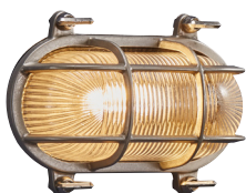
Helford 49031055 Nickel | Brass Excl. E27 | Max. 12.5W H: 12,5 cm | W: 19 cm
